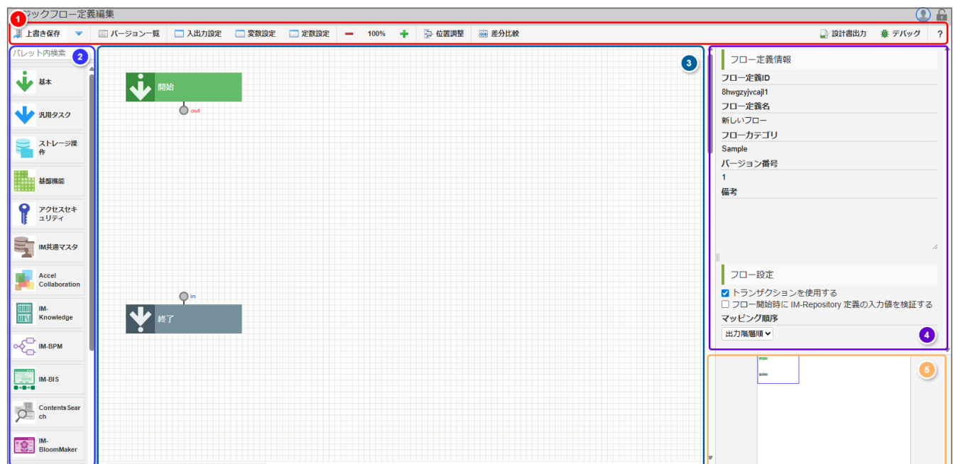
図：ロジックフロー定義編集画面の詳細
