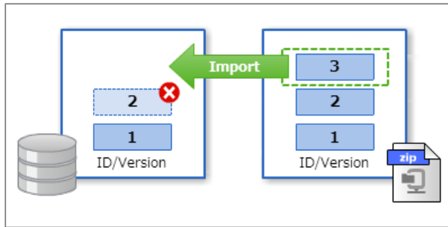
図: 論理削除状態のバージョンも含めて、新規バージョンのみインポート
