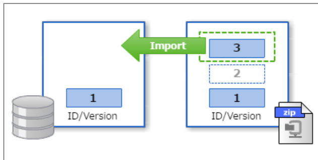
図: 一部バージョンが含まれないデータのインポート処理
