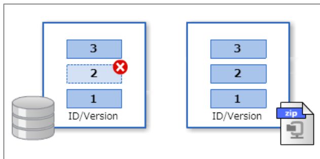
図: インポートが行われない場合（インポート先に論理削除状態のバージョンがある）
