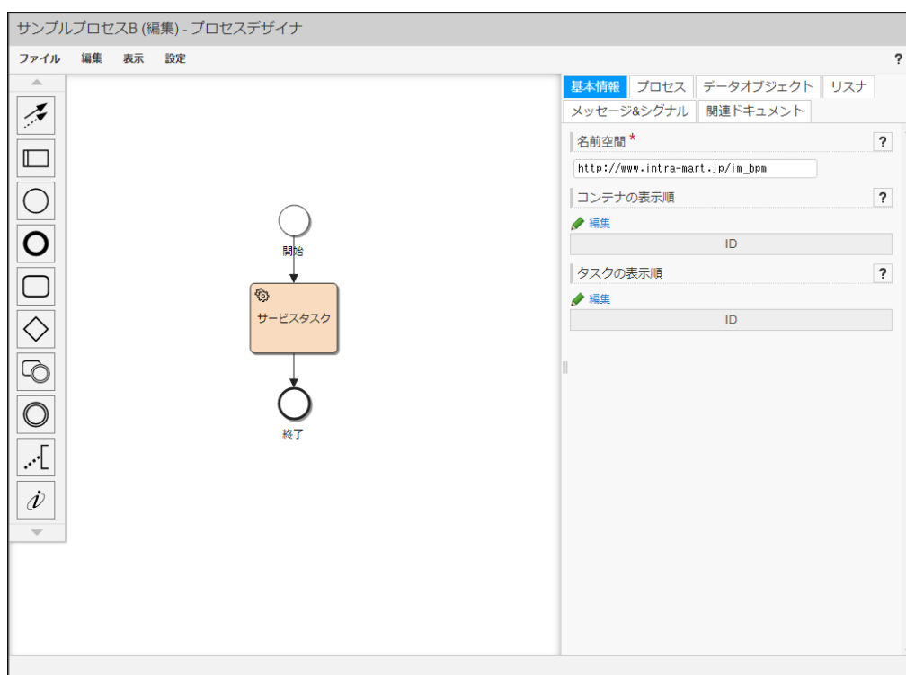
図：「プロセスエディタ」
