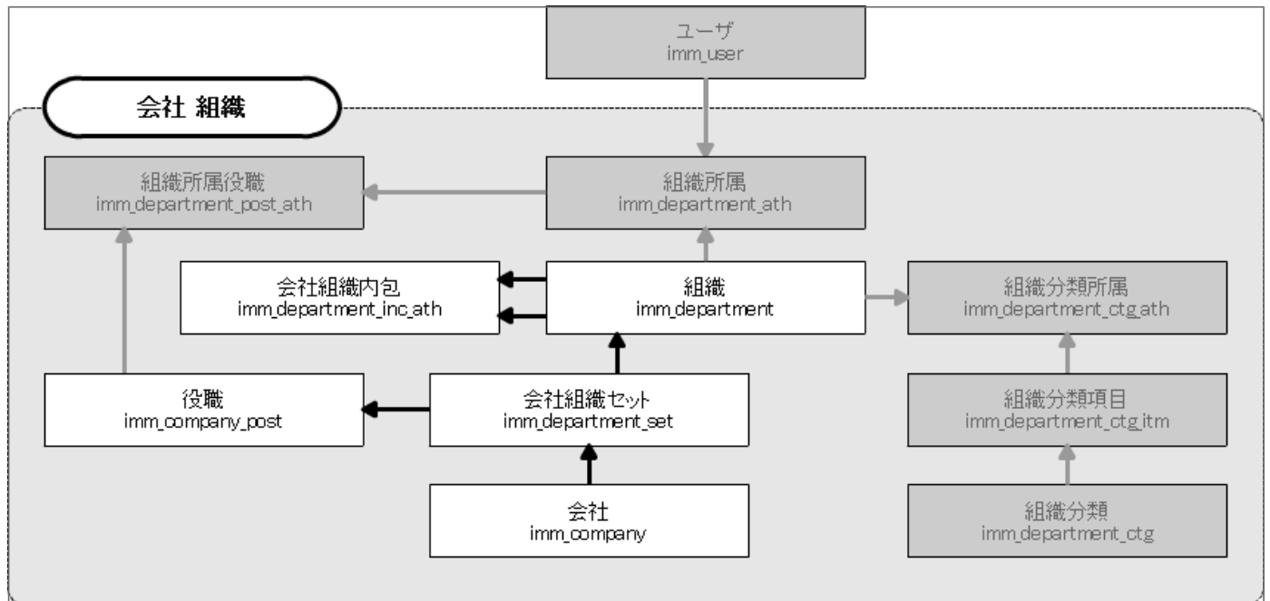
【図：会社・組織の構成に関するER図】
