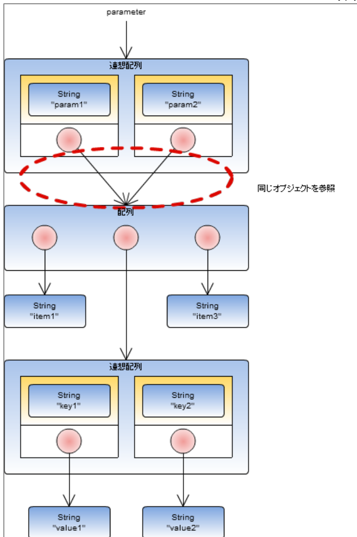
同一インスタンスを参照しているパラメータ（イメージ図）
