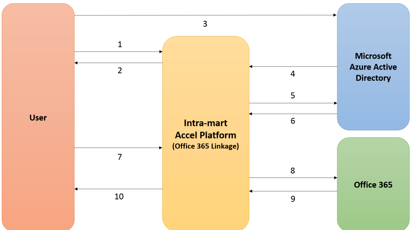
Office 365 連携のフロー図
