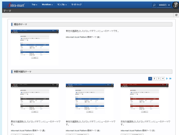
「テーマ」画面
