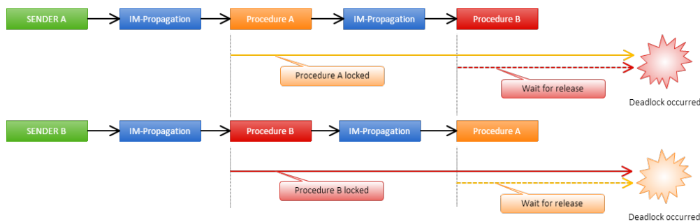
図 デッドロック発生時の例
