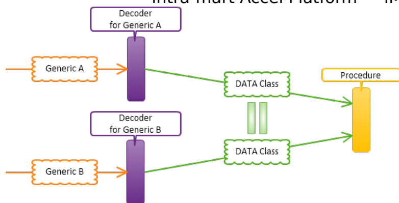
図 「受信側のデータ変換クラス（Decoder）」 「受信側のデータ処理クラス（Procedure）」の関係
