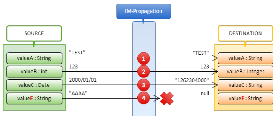
図 クラスの復元イメージ
