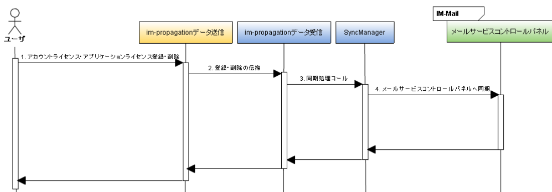
図 UserListener シーケンス図
