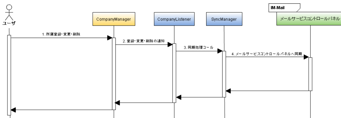
図 CompanyListener シーケンス図
