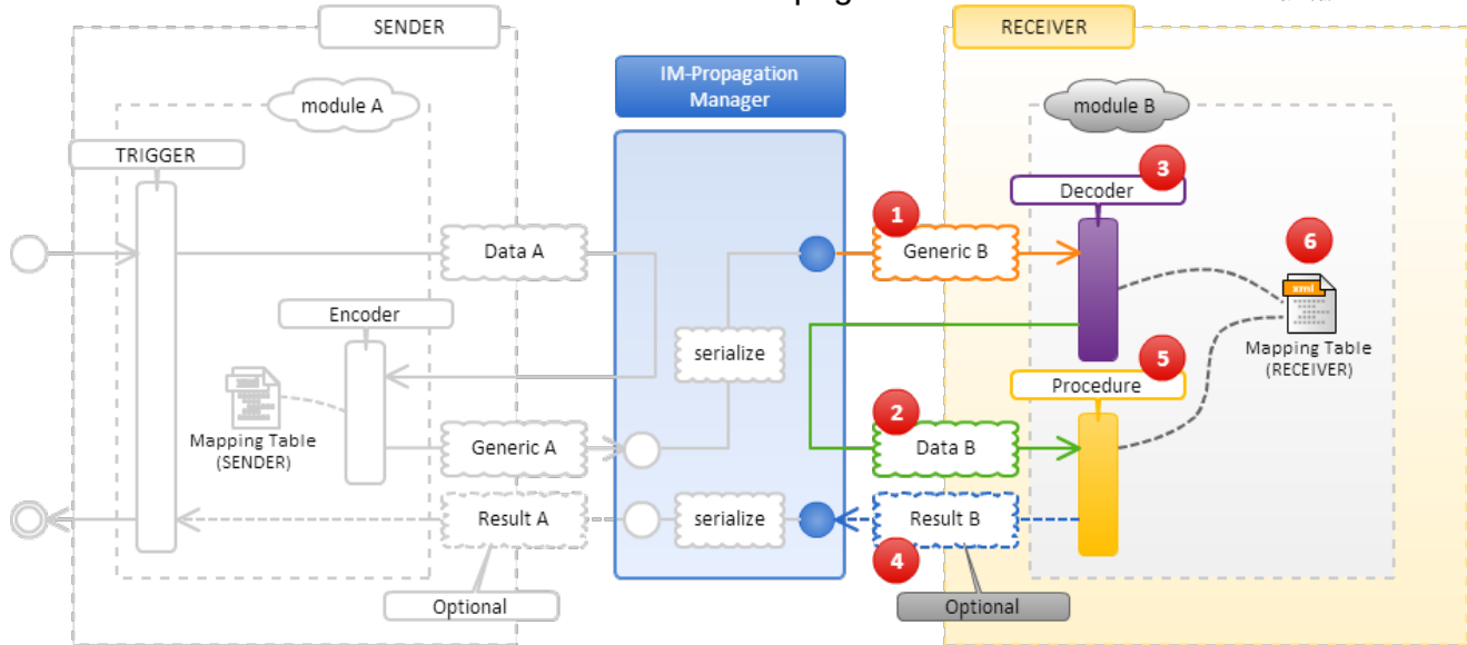
図 受信側の処理
