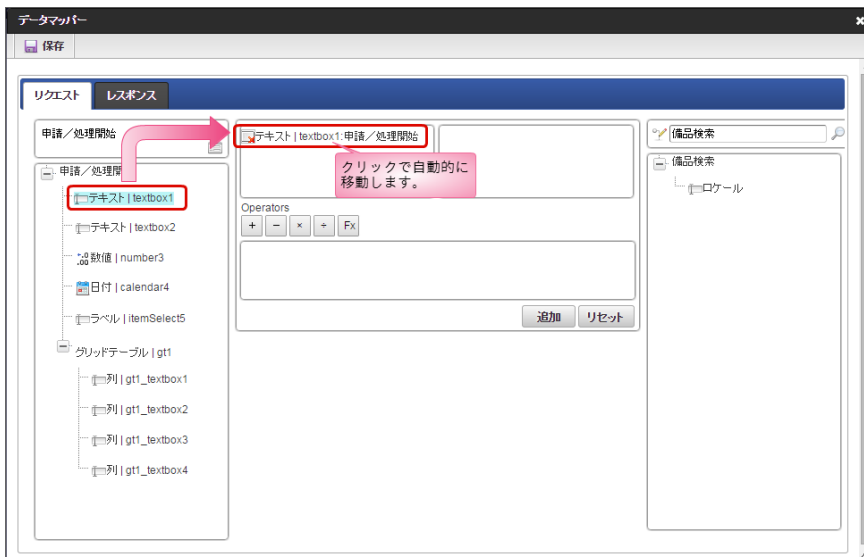
15. 右側のツリーから項目をクリックすると、マッピング対象の枠に追加されます。
