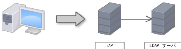
図 LDAP 構成
