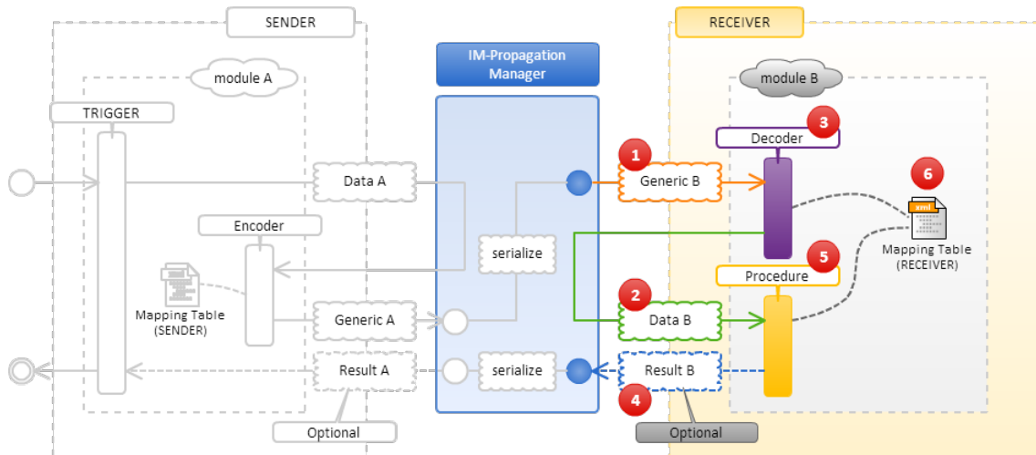
図 受信側の処理
