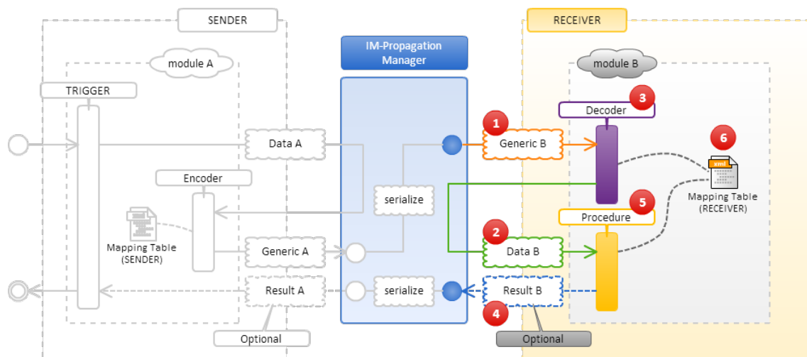
図 受信側の処理
