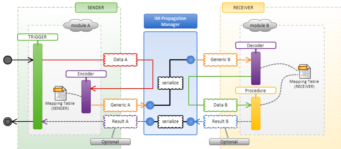
図 データの流れ
