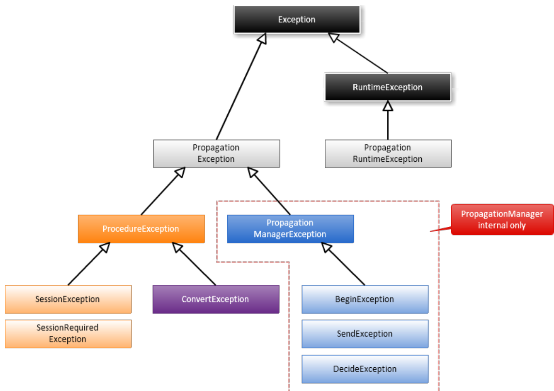
図 例外クラスの関係
