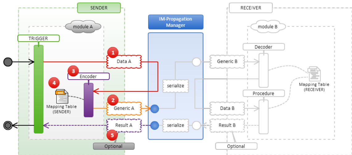
図 送信側の処理
