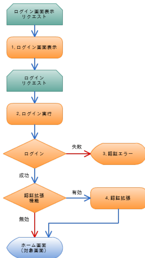
図 一般ユーザのログインリクエストフロー
