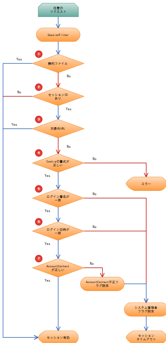
図 セッションタイムアウト検出フロー
