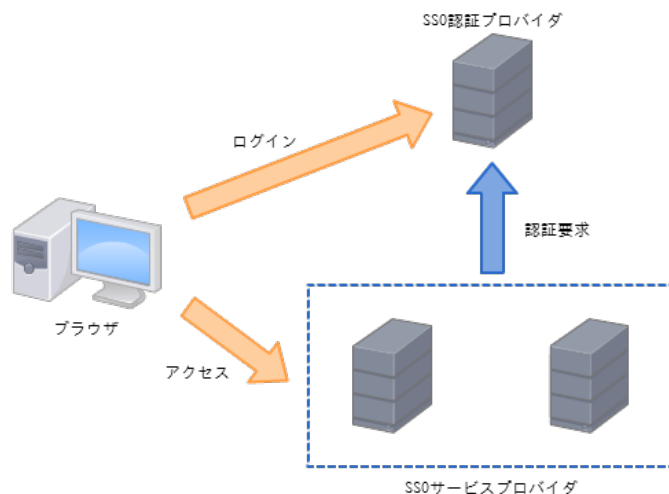
図 SSOの構成
