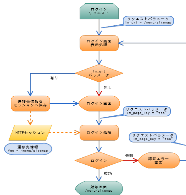
図 遷移先情報の持ちまわり
