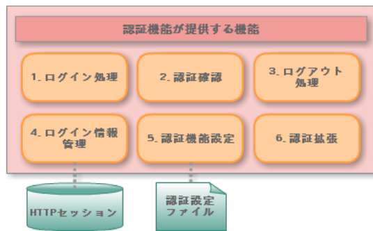
図 認証機能が提供する機能
