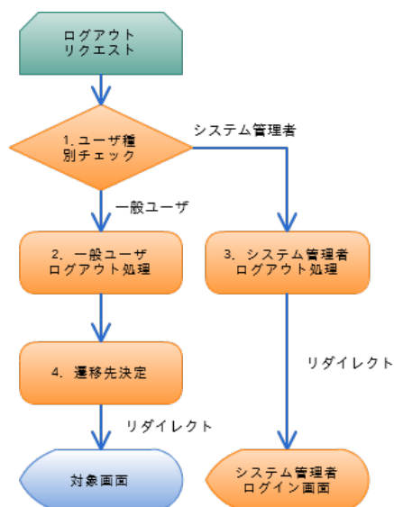
図 ログアウト処理フロー
