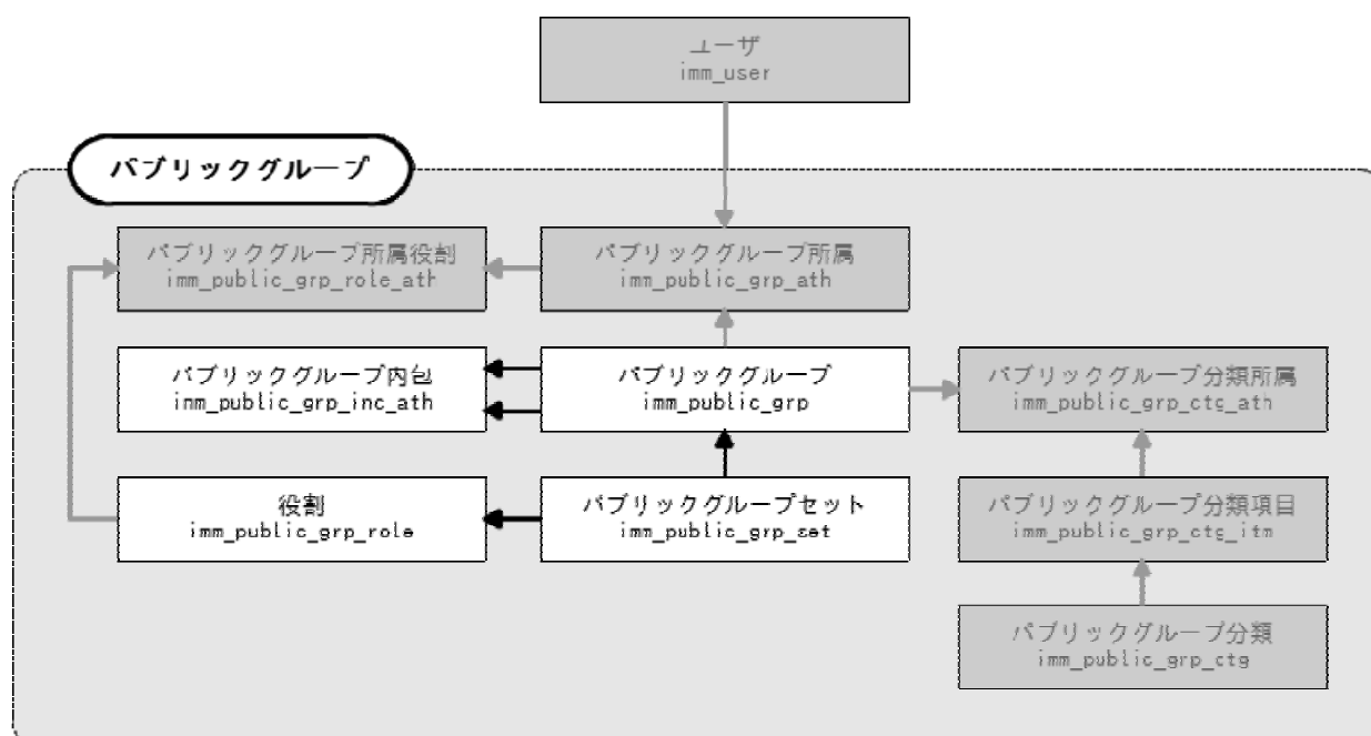
図 2-6 パブリックグループの構成に関連する ER 図
