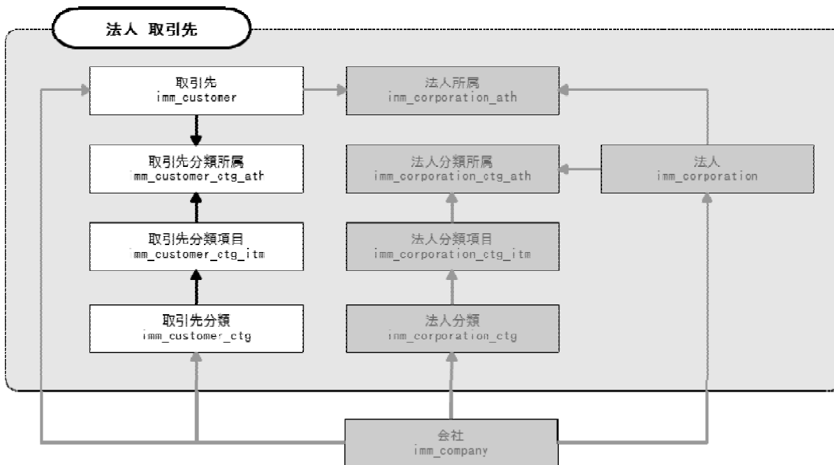
図 2-13 取引先分類に関するER図
