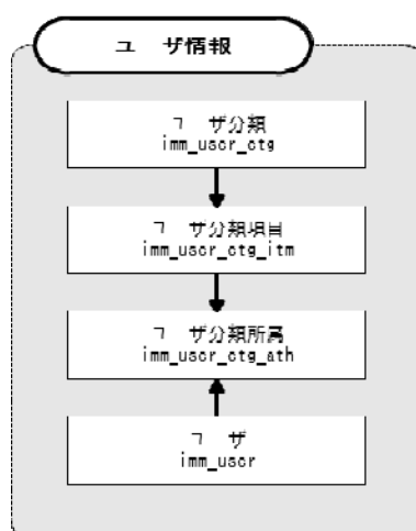
図 2-1 ユーザ及びユーザ分類関連のER図
