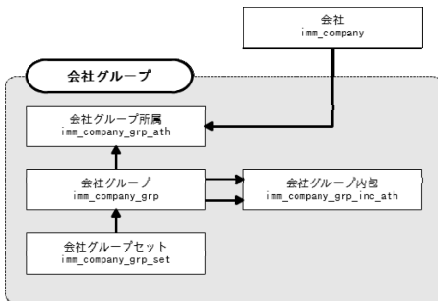
図 2-5 会社グループの構成に関連する ER 図
