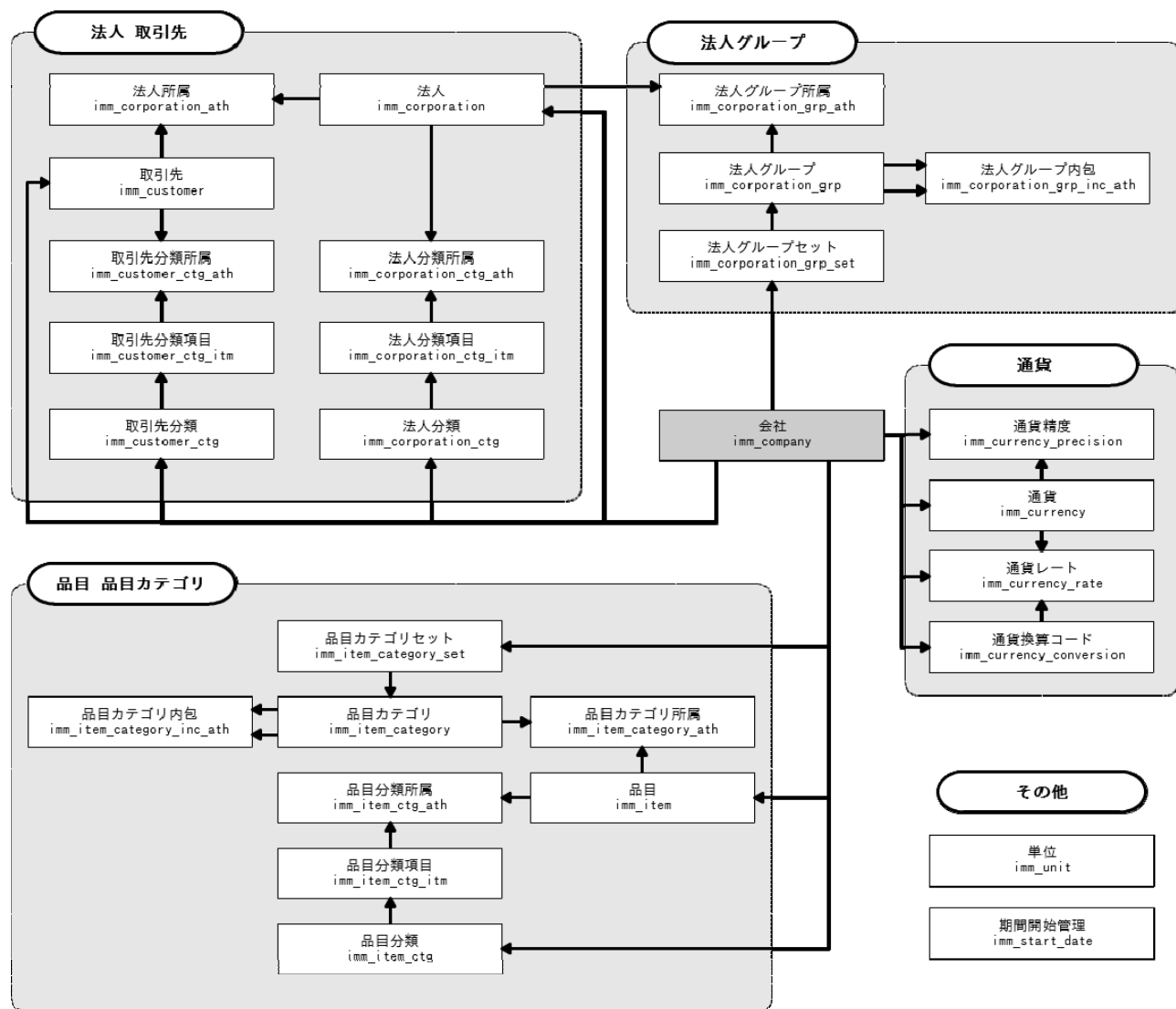
図 1-1 データ構成(全体)
