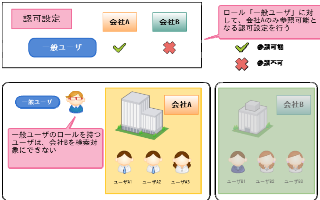
図 1-17 認可の制御イメージ
