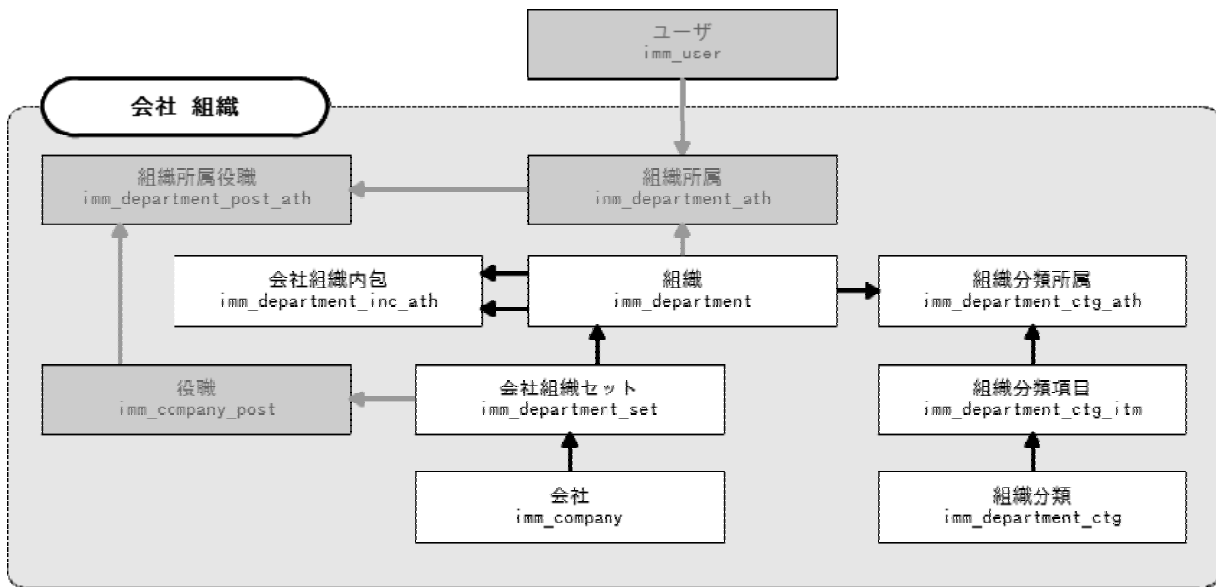
図 2-4 会社・組織の分類に関連する ER 図
