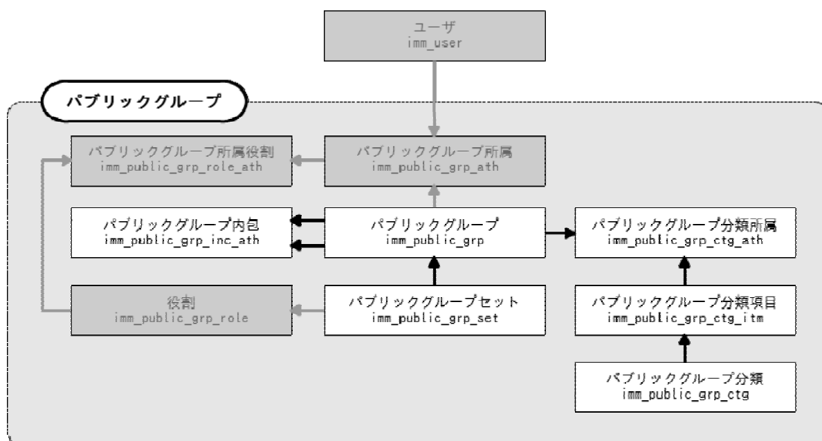
図 2-8 パブリックグループの分類に関連するER図
