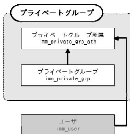
図 2-9 プライベートグループに関連する ER 図
