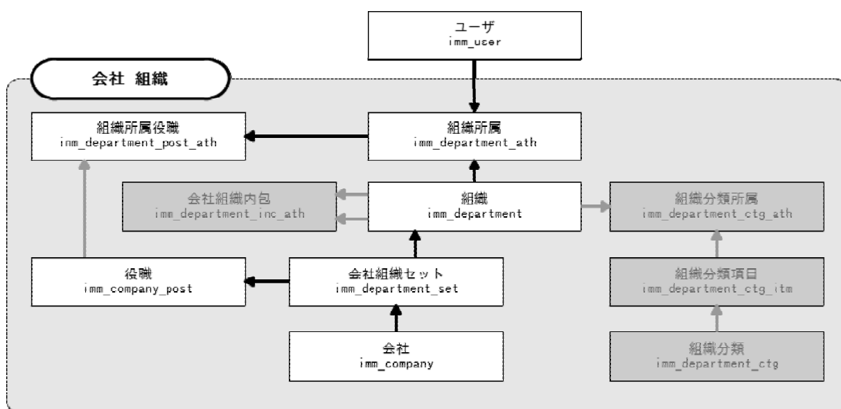
図 2-3 会社・組織とユーザの所属に関連する ER 図
