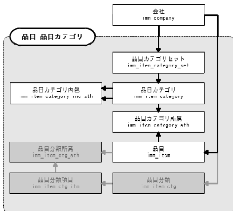
図 2-10 品目カテゴリに関連する ER 図
