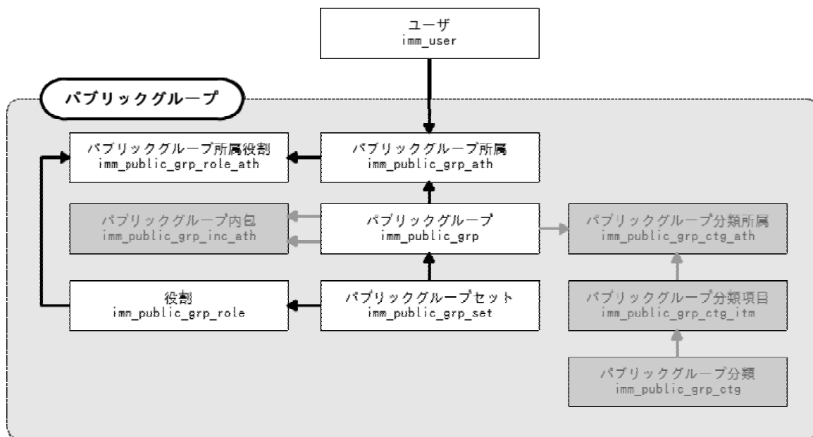
図 2-7 パブリックグループとユーザの所属に関連する ER 図
