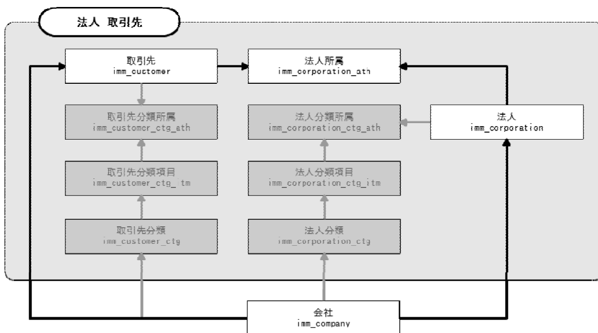
図 2-12 法人に関連する ER 図
