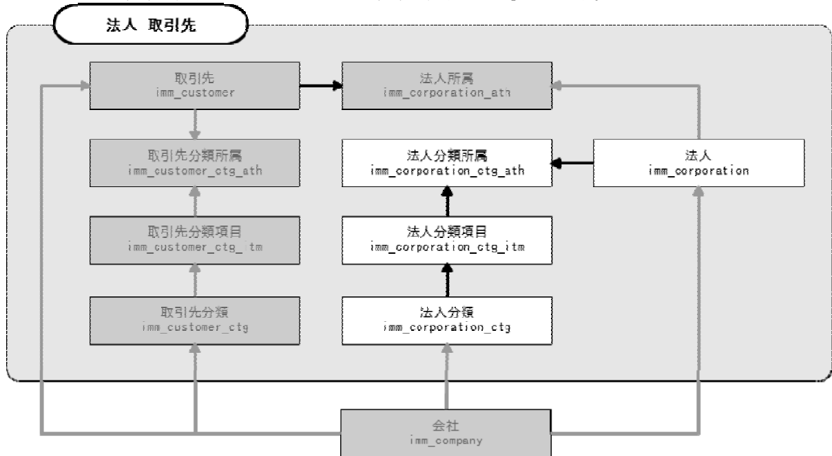
図 2-14 法人分類に関するER図
