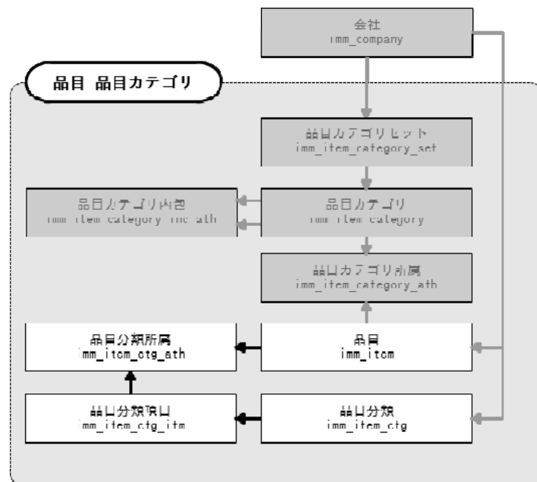
図 2-11 品目分類に関連するER図
