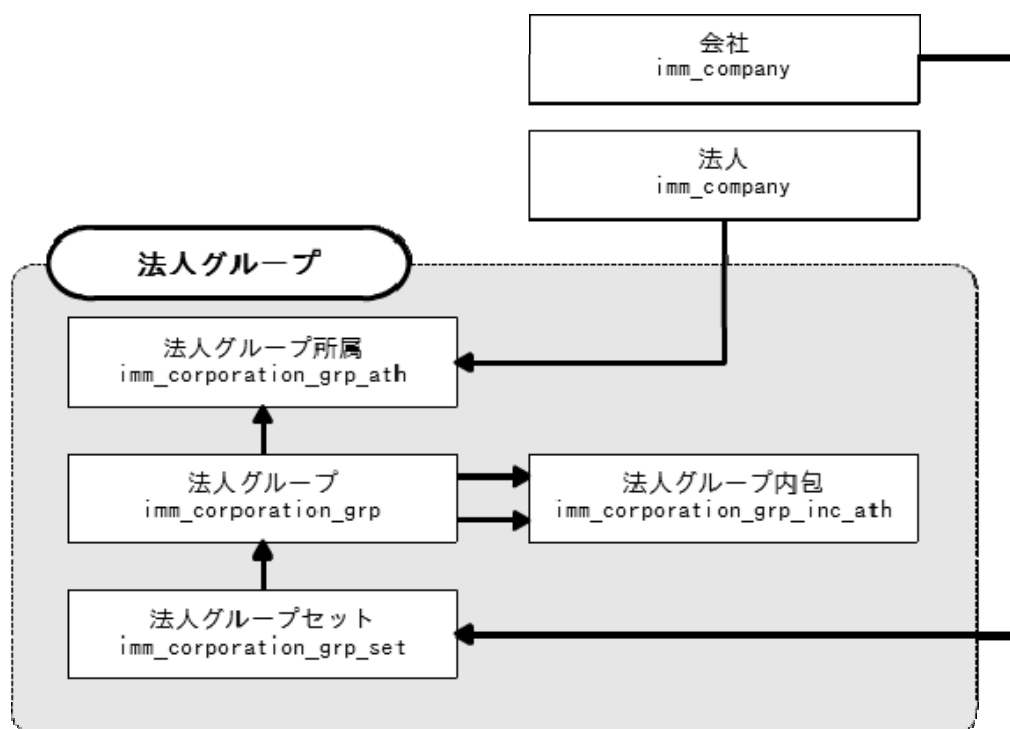
図 2-15 法人グループの構成に関連する ER 図
