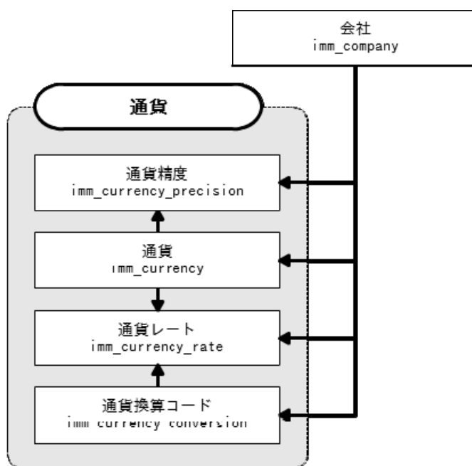
図 2-16 通貨に関するER図
