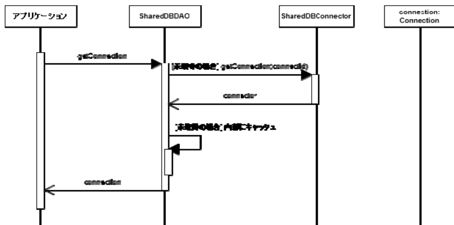
図 5-9 Connection の取得 (SharedDBDAO)
