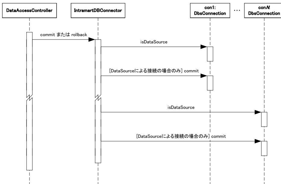
図 5-36 コミットまたはロールバック (IntramartDBConnector)
