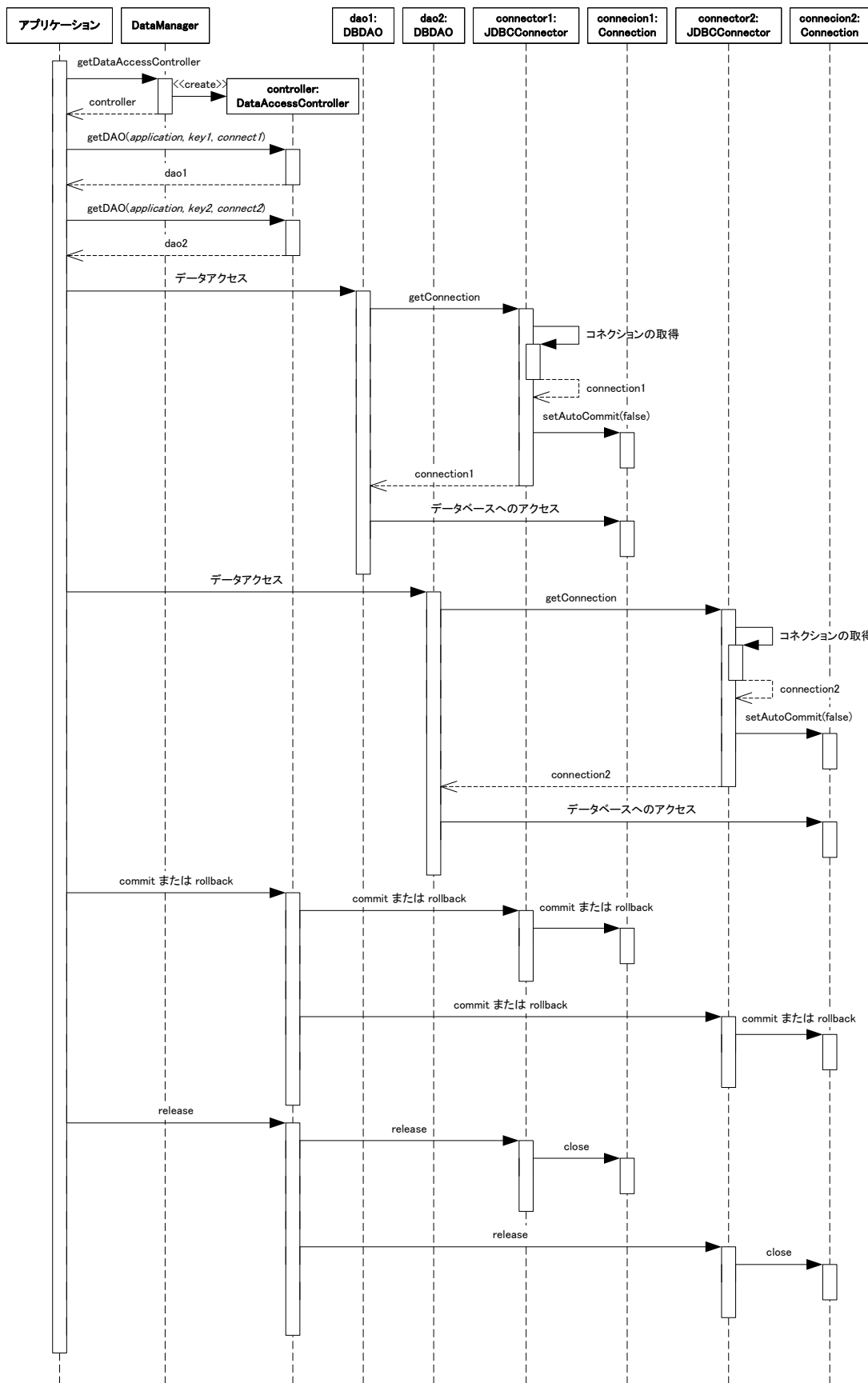
図 5-48 複数 DAO、複数コネクション
