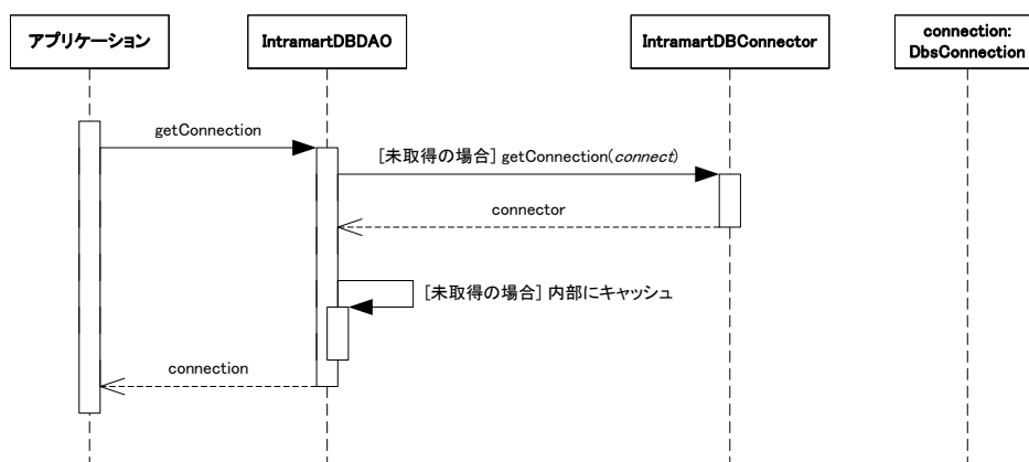
図 5-11 Connection の取得 (IntramartDBDAO)
