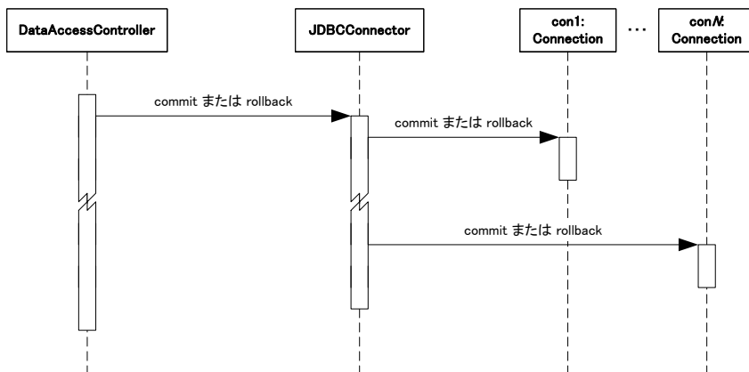
図 5-23 コミットまたはロールバック (JDBCConnector)
