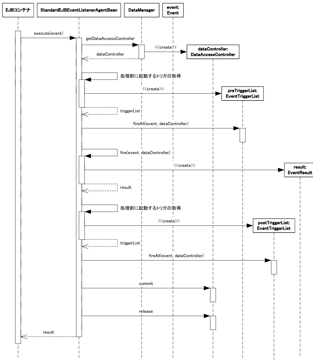
図 4-26 StandardEJBEventListener のトランザクション
