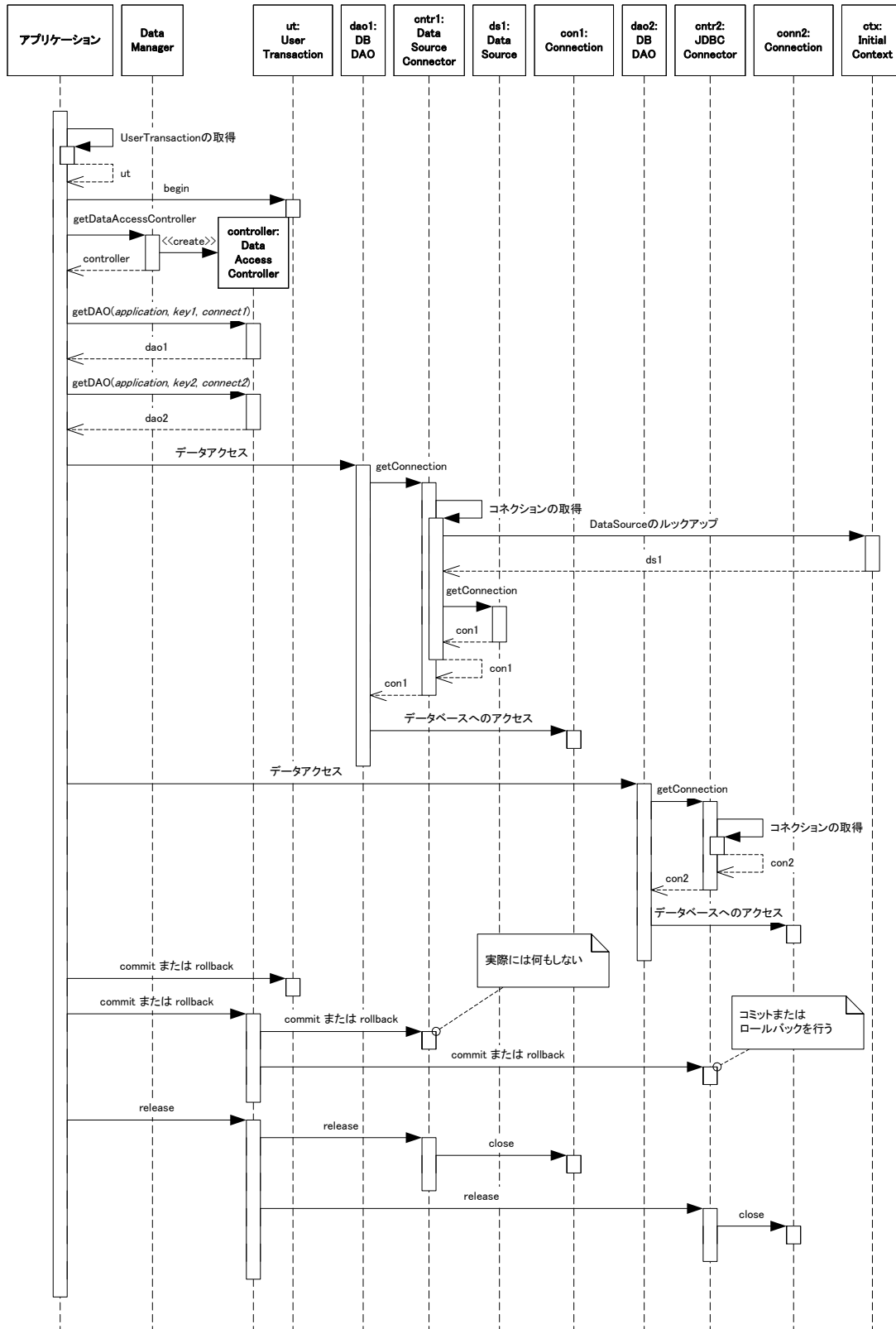
図 5-50 複数 DAO、複数コネクション (DataSource と JDBC の併用)
