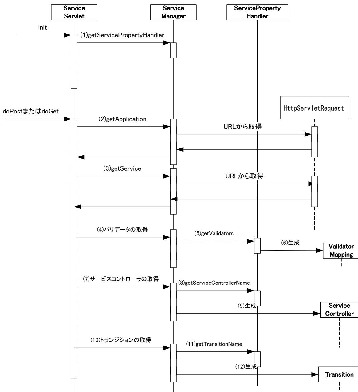
図 3-9 サービスフレームワーク(準備)
