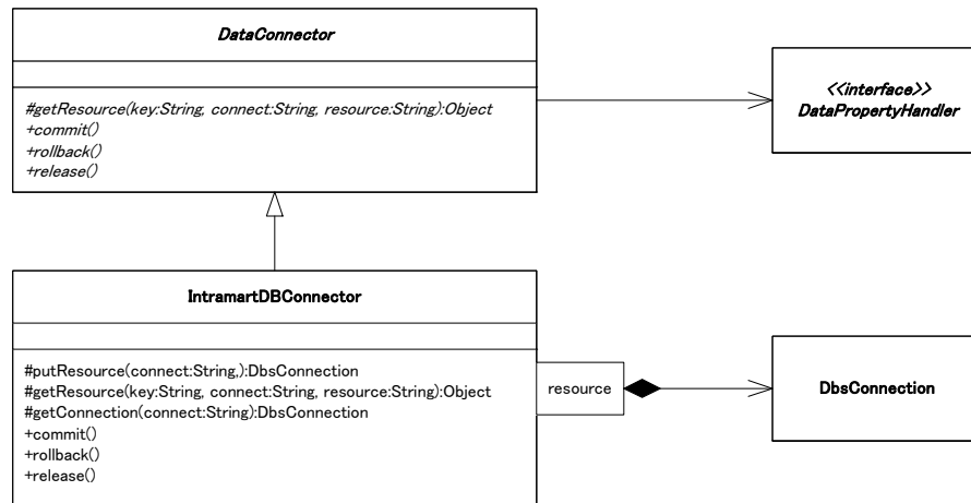
図 5-34 IntramartDBConnector の構造
