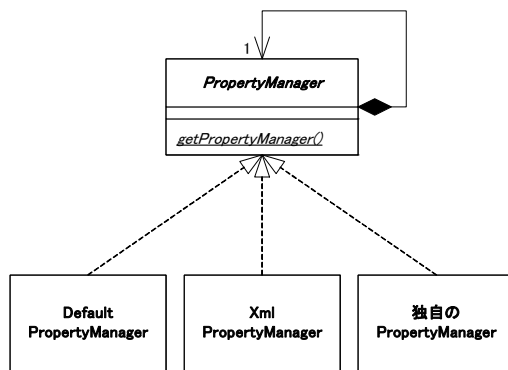
図 8-4 PropertyManager の構造
