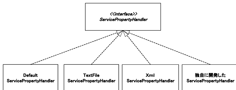
図 3-6 ServicePropertyHandler
