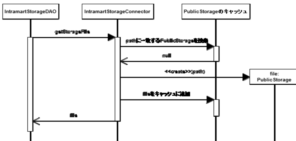
図 5-38 PublicStorage の取得
