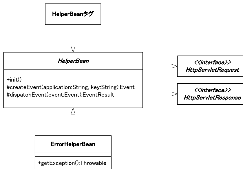
図 3-24 HelperBean の構成
