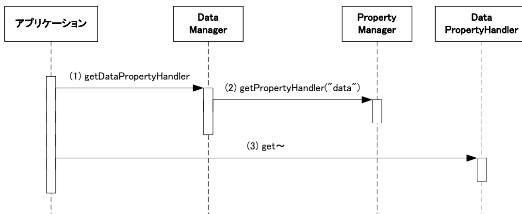
図 5-41 DataPropertyHandler の取得
