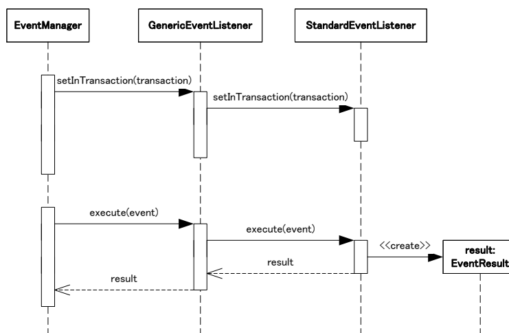
図 4-14 GenericEventListener の動作
