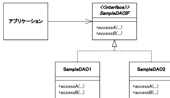
図 5-14 DAOIF の利用
