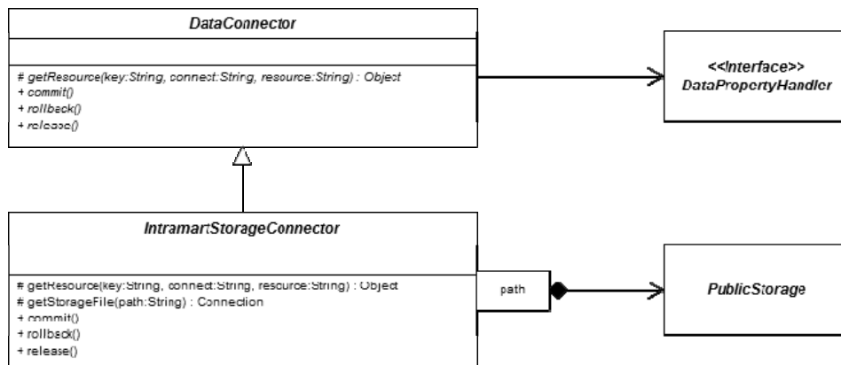
図 5-37 IntramartStorageConnector の構造
