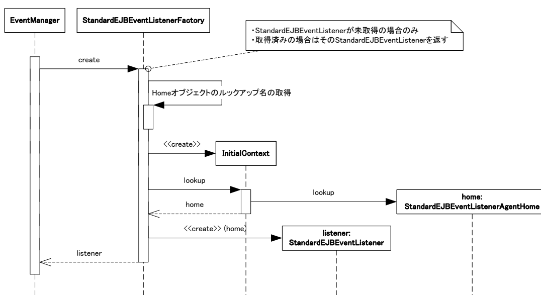
図 4-10 StandardEJBEventListener の生成
