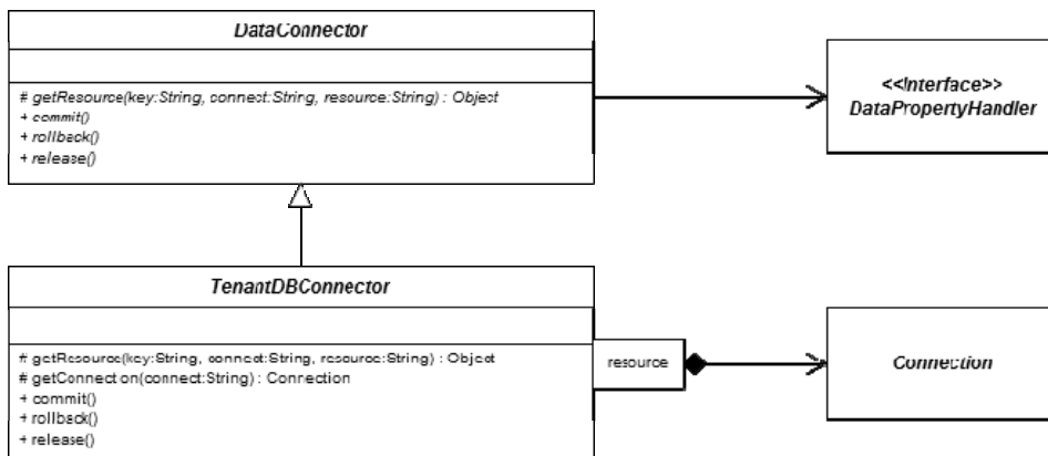
図 5-27 TenantDBConnector の構造
