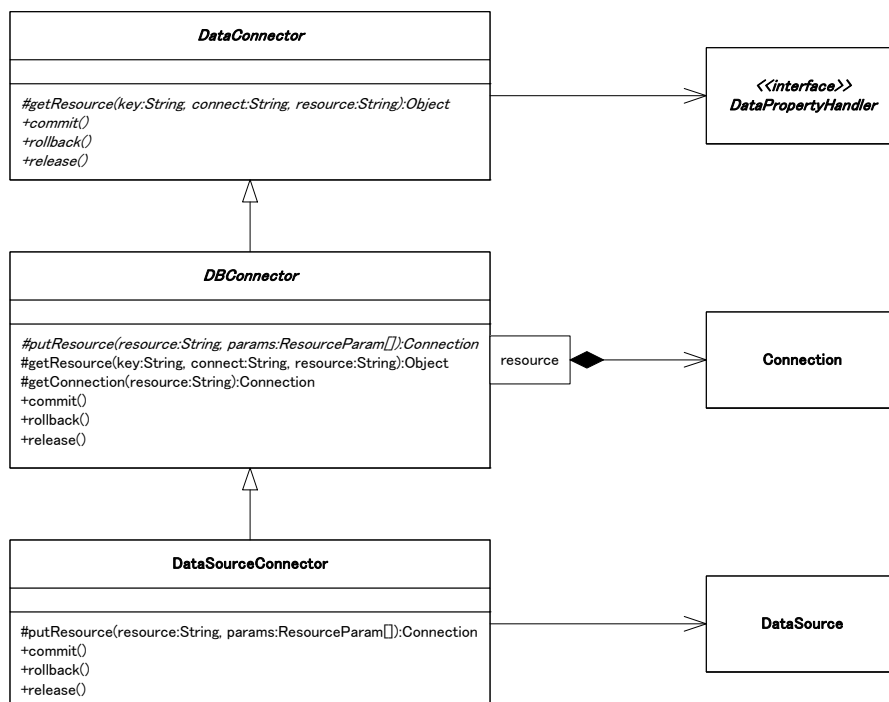
図 5-24 DataSourceConnector の構造
