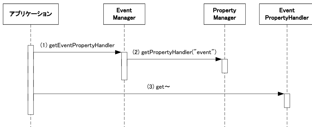
図 4-22 EventPropertyHandler の取得
