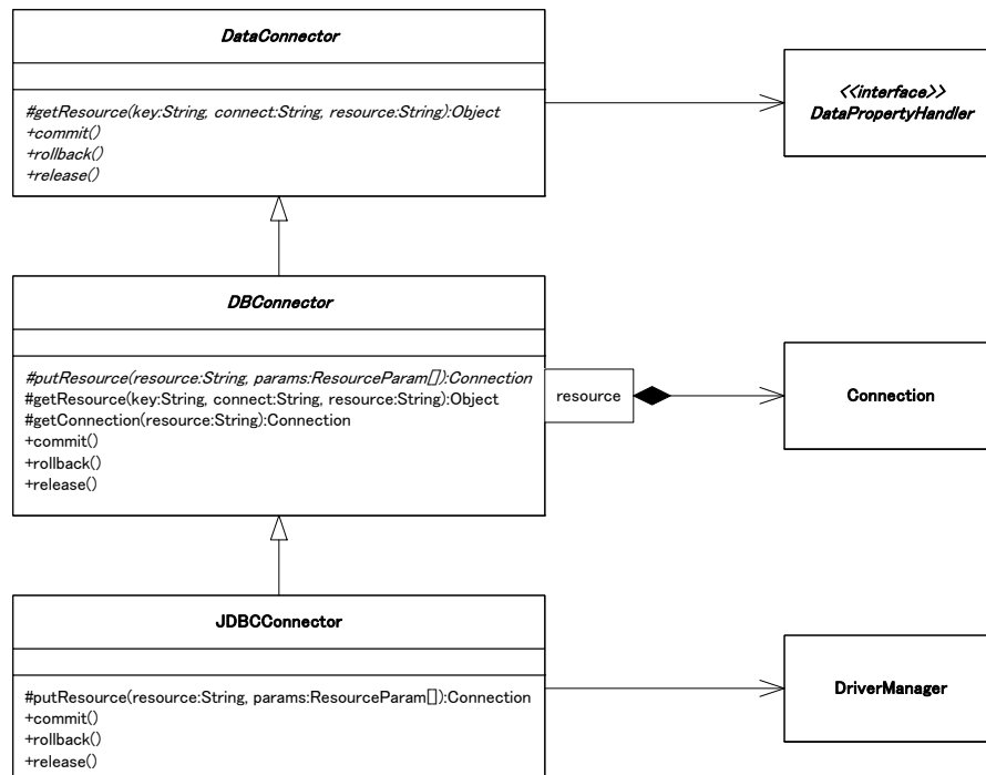
図 5-21 JDBCConector の構造
