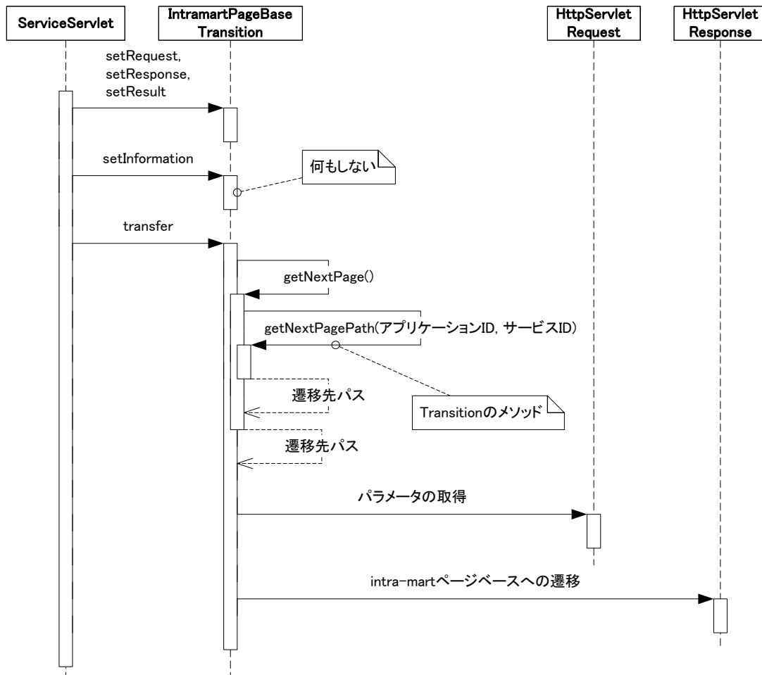
図 3-23 IntramartPageBaseTransition の動作
