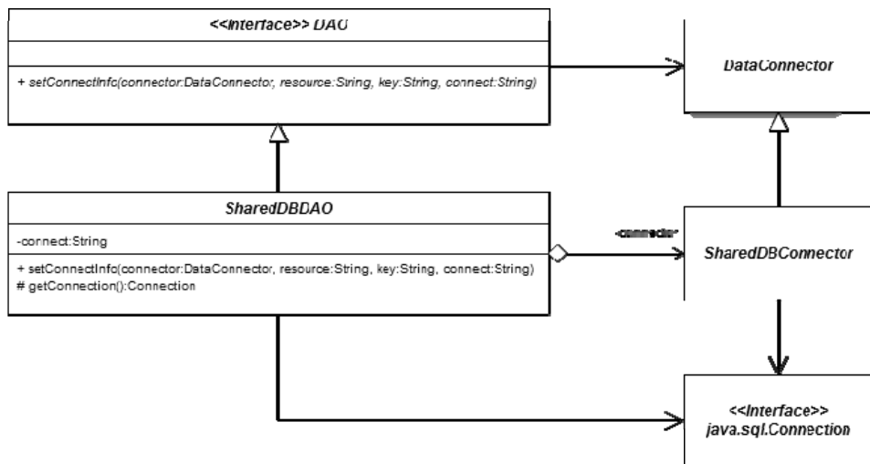
図 5-8 SharedDBDAO の構造
