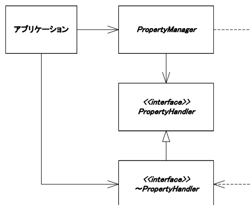
図 8-1 PropertyHandler の構成
