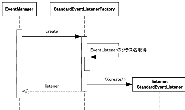
図 4-8 StandardEventListener の生成
