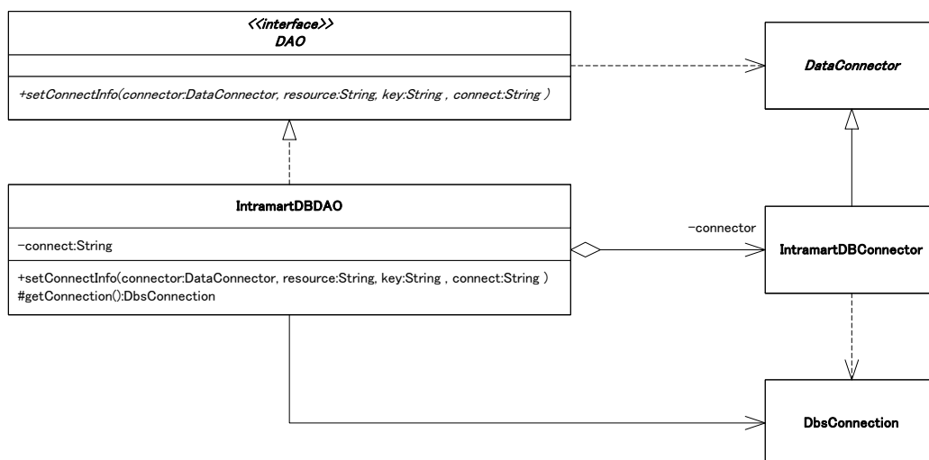
図 5-10 IntramartDBDAO の構造
