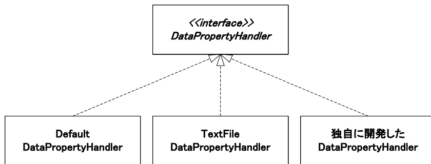
図 5-40 DataPropertyHandler
