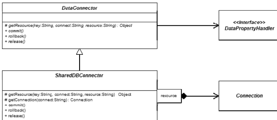
図 5-31 SharedDBConnector の構造
