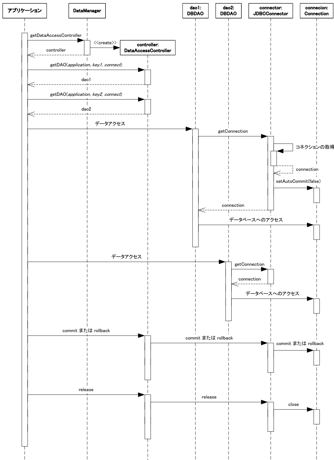
図 5-47 複数 DAO、単一コネクション
