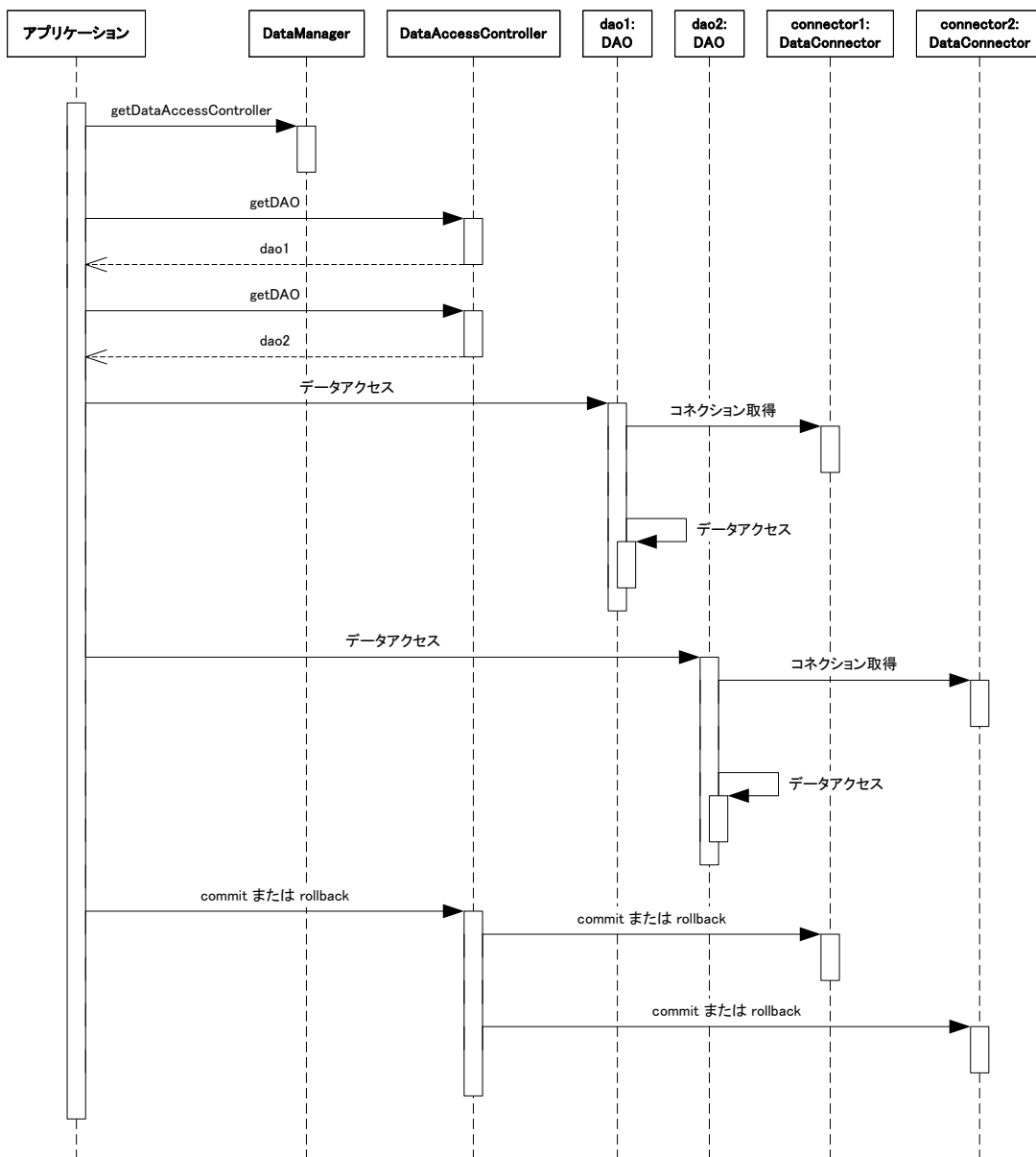
図 5-44 DataAccessController によるトランザクション管理
