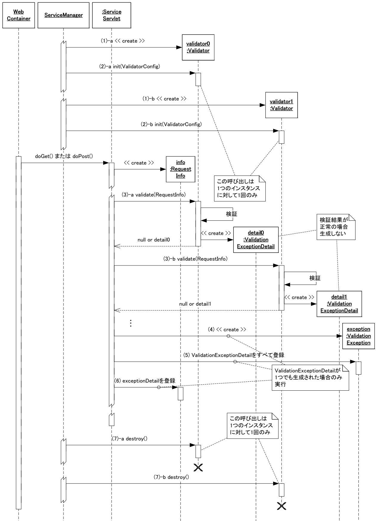
図 3-13 Validator の管理
