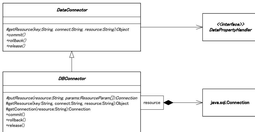
図 5-18 DBConnector の構造
