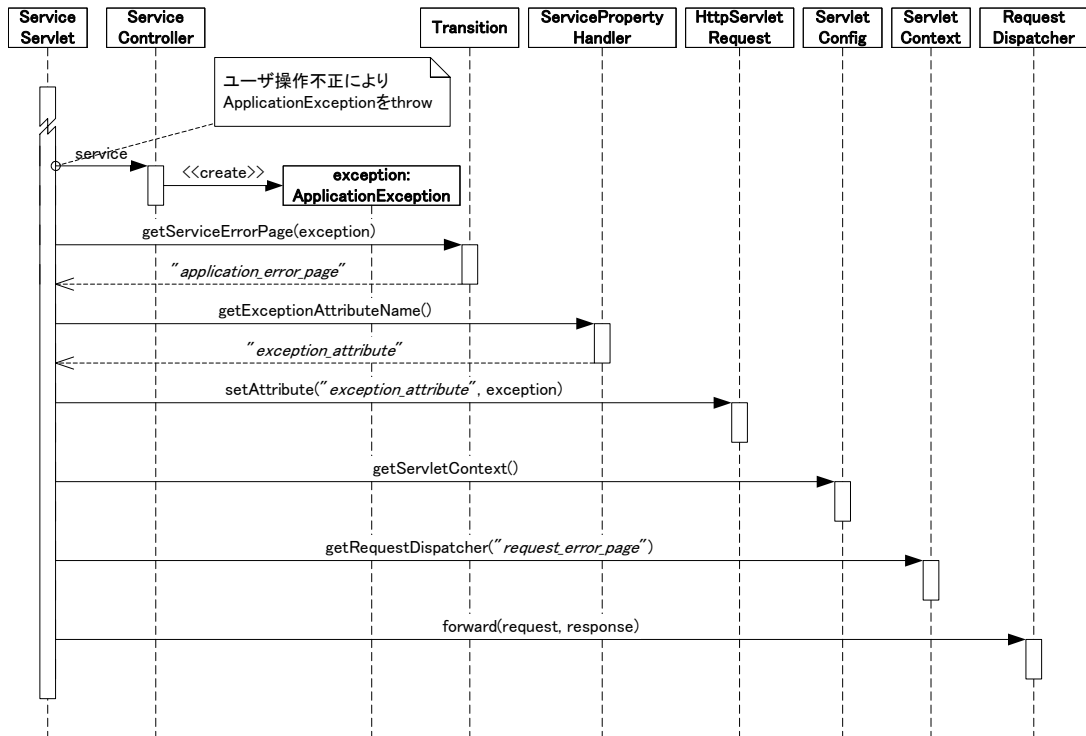
図 3-29 ApplicationException 発生時
