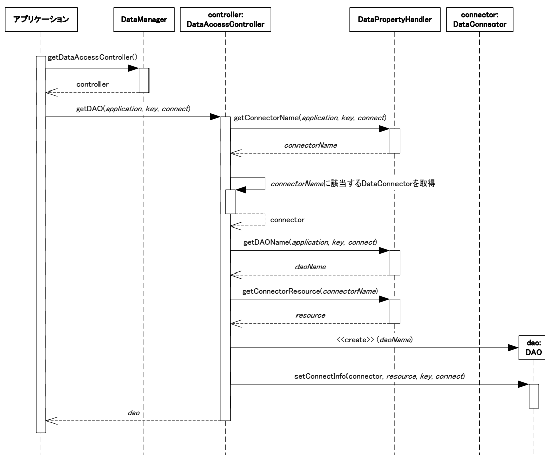
図 5-15 DAO の取得
