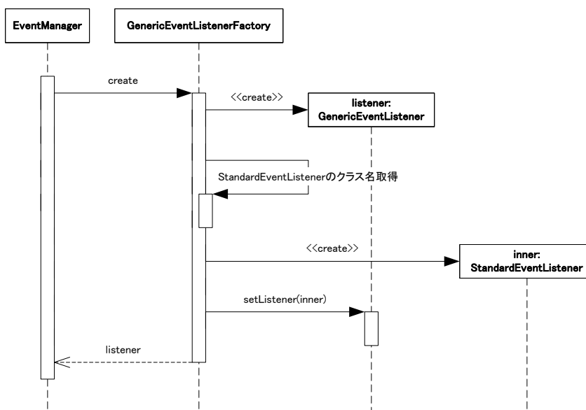
図 4-9 GenericEventListener の生成
