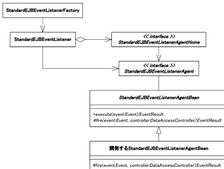
図 4-15 StandardEJBEventListener の構造
