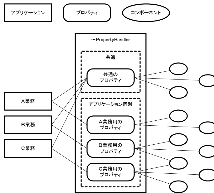
図 2-3 PropertyHandler
