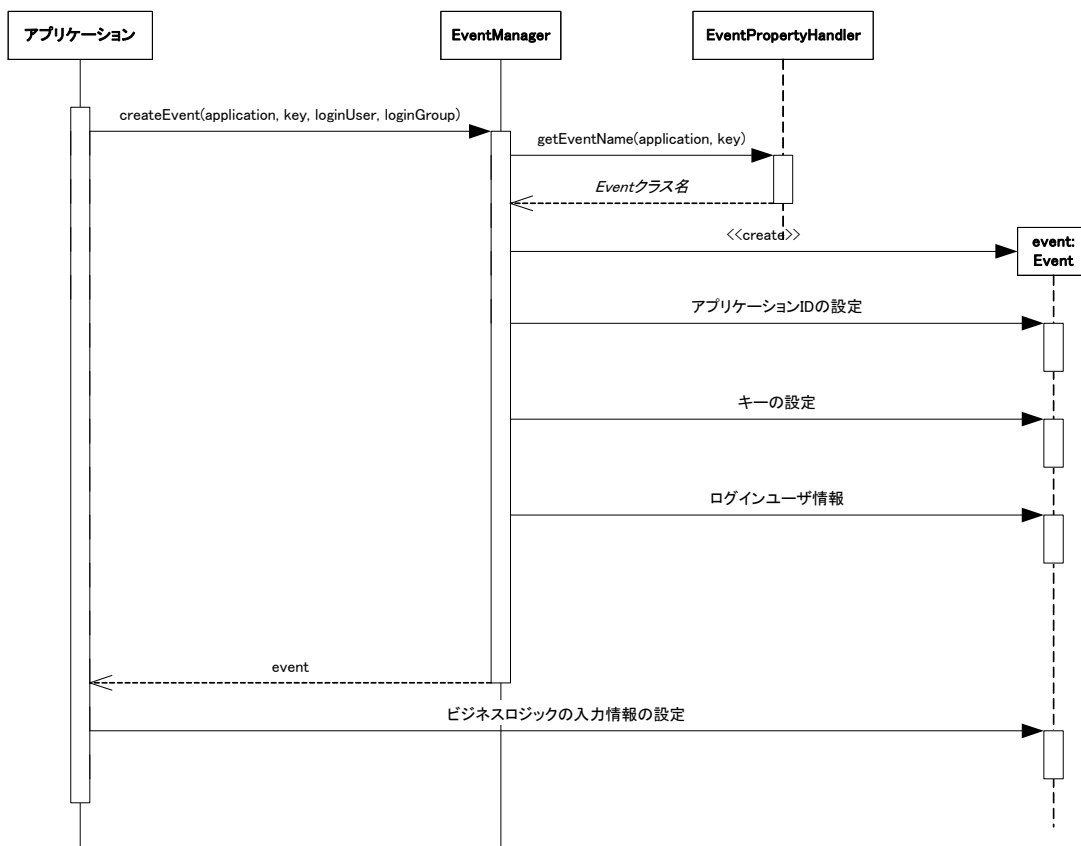
図 4-3 Event の生成
