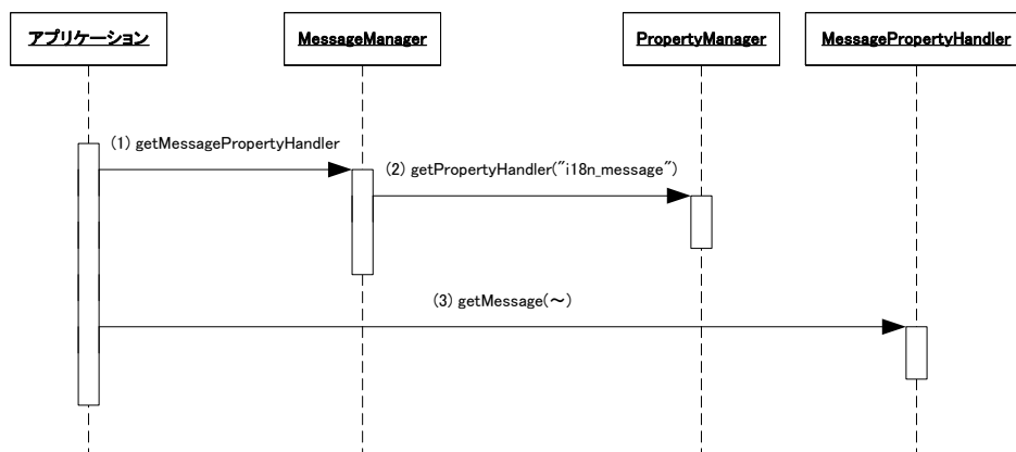
図 6-4 MessagePropertyHandler の取得
