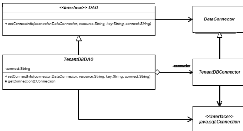
図 5-6 TenantDBDAO の構造
