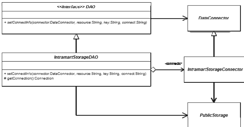
図 5-12 IntramartStorageDAO の構造
