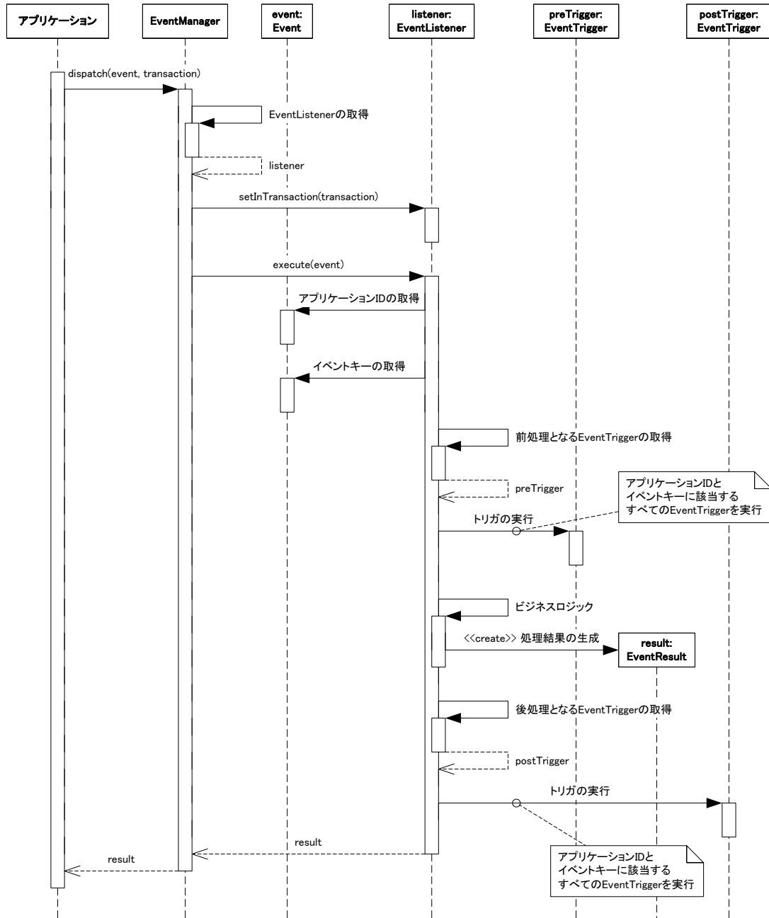
図 4-12 EventListener の概要
