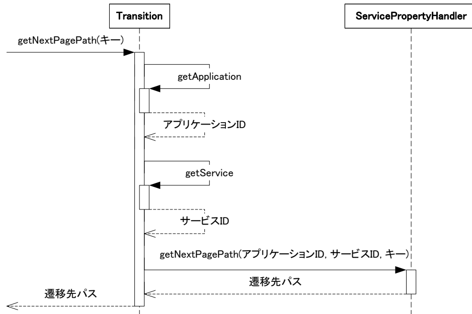
図 3-21 Transition の getNextPathPage(キー付)
