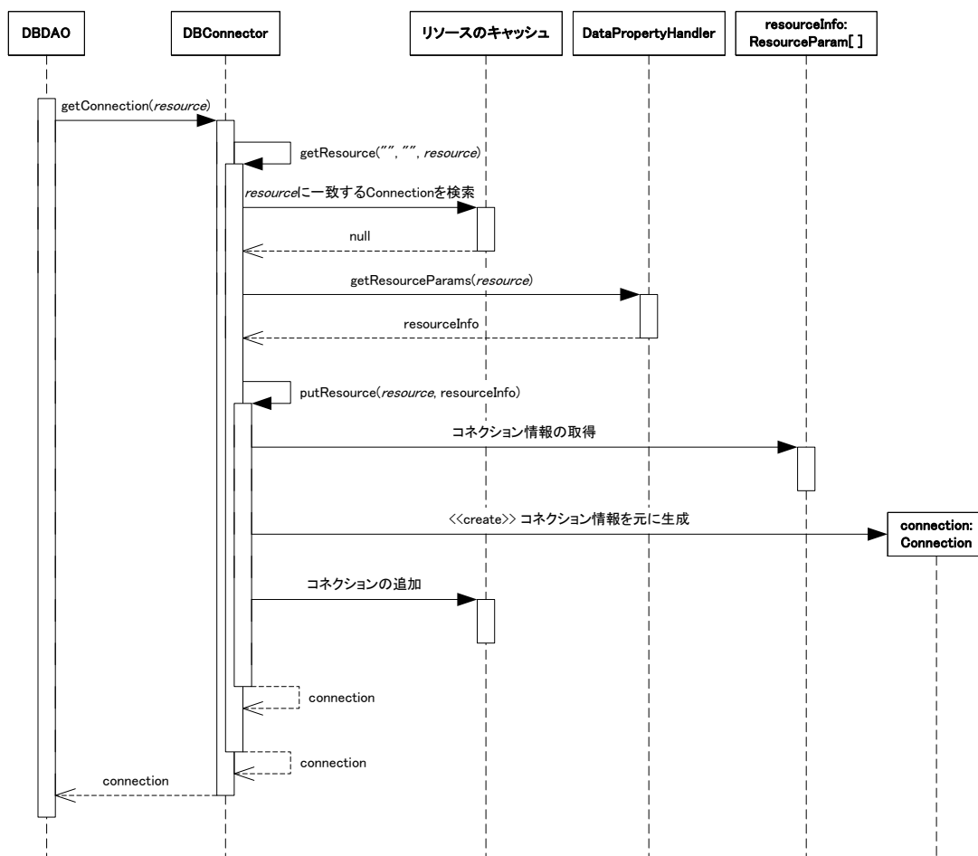
図 5-20 DBConnector から Connection を取得 (新規)
