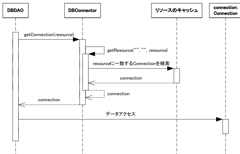
図 5-19 DBConnector から Connection を取得 (取得済)
