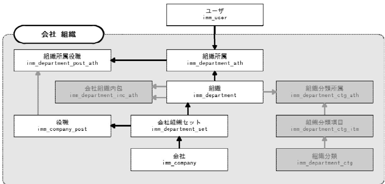
図 2-3 会社・組織とユーザの所属に関連する ER 図
