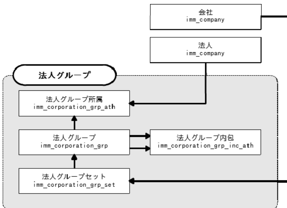
図 2-15 法人グループの構成に関連する ER 図
