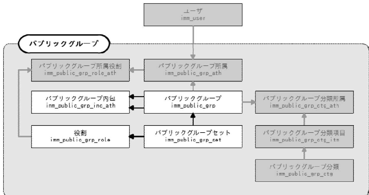
図 2-6 パブリックグループの構成に関連する ER 図
