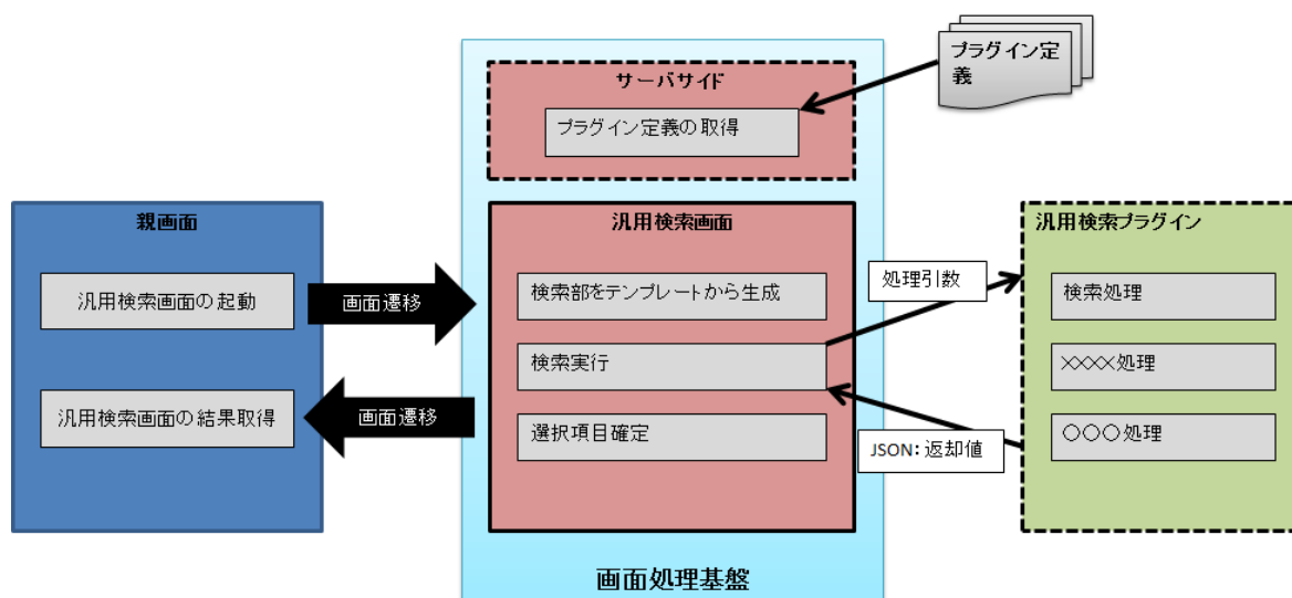
図 2-1 汎用検索画面タブの動作概要
